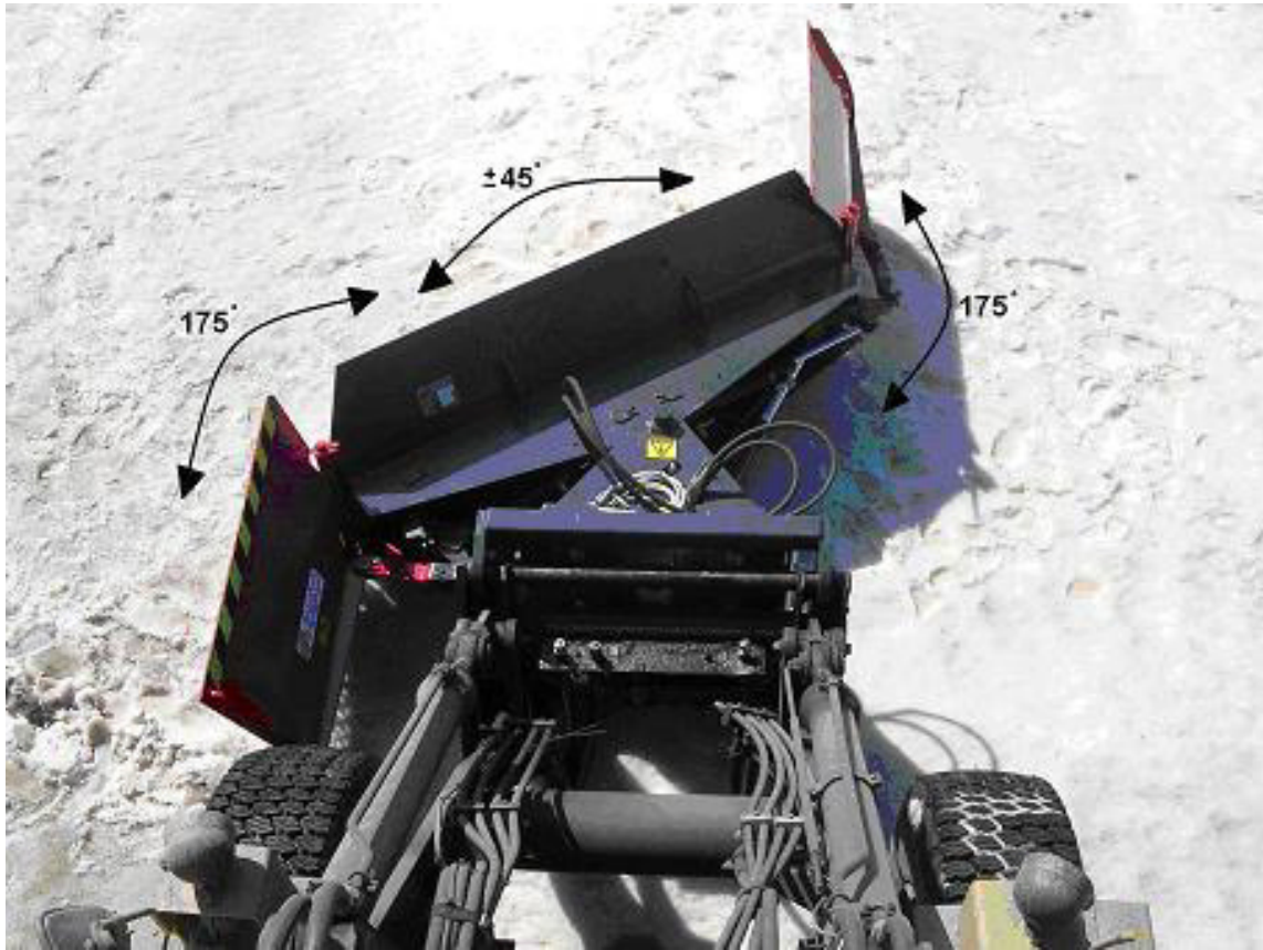
Multi 3000 nähtynä ohjaamosta: Uusi vahvempi eturunko ja suurempi kääntökulma.
